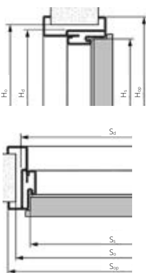
DRZWI WAHADŁOWE OŚCIEŻNICA DREWNIANA STAŁA
