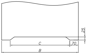
podcięcie wentylacyjne w skrzydłach bezprzylgowych - dopłata powierzchnie fornirowane 50/61,50 - dopłata powierzchnie syntetyczne/malowane 35/43,05
