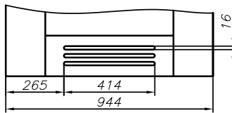
skrzydło „90” ze szczeliną wentylacyjną
