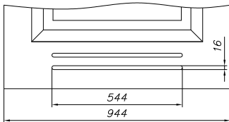
skrzydło „90” ze szczeliną wentylacyjną
