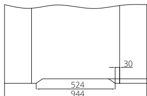
skrzydło „90” z podcięciem wentylacyjnym
