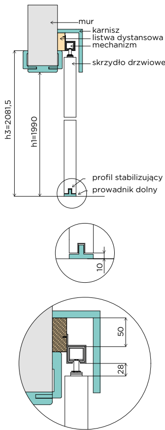
OPASKA 80 mm H1=1990 mm
