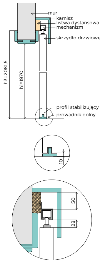
OPASKA 100 mm H1=1970 mm
