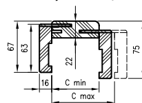
Przekrój TUN z kątem T63
